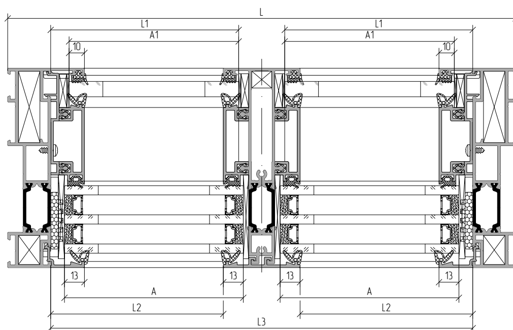
Горизонтальные сечения
