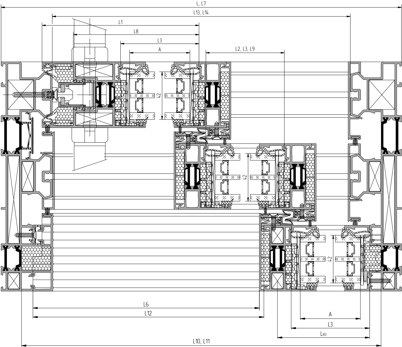
Горизонтальные сечения. Исполнение 1
