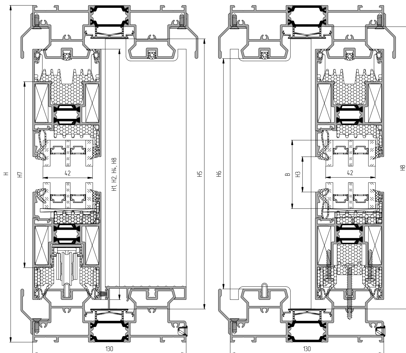
Вертикальные сечения
