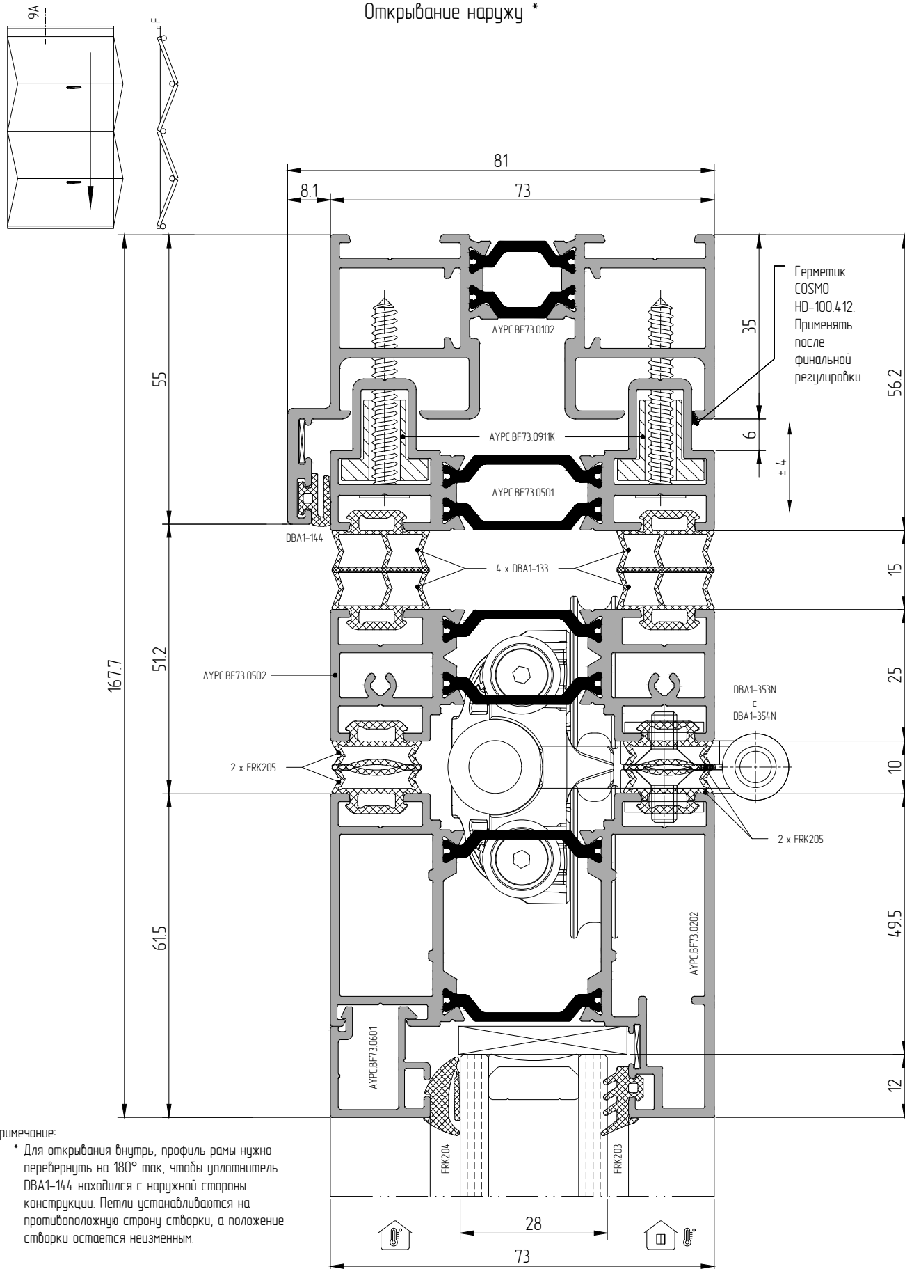
Сечение 9 – Фурнитурный узел F А.2 – Стык штульпа АУРС.ВF73.0502 и регулировочного профиля. Стандартная створка АУРС.ВF73.0202
