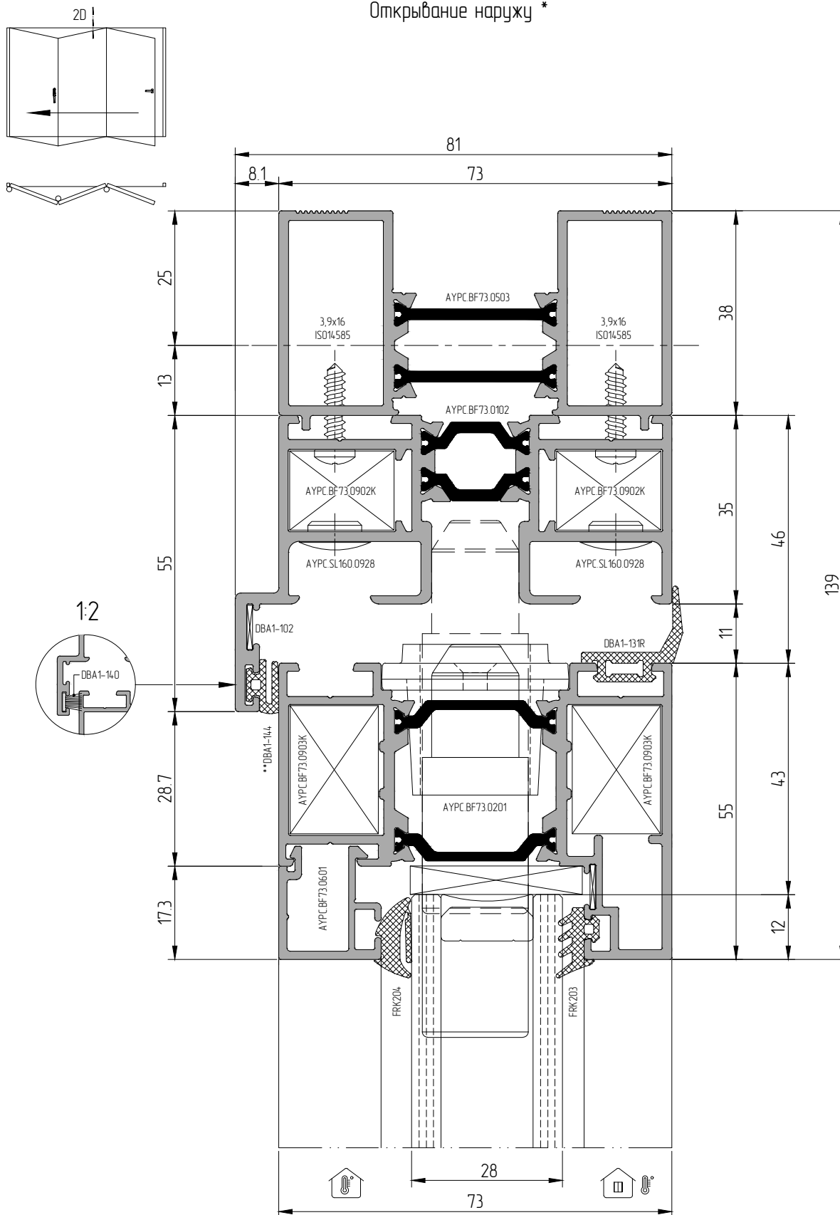
Сечение 2 – Верхний узел D.1 – Рама АУРС.ВF73.0102 со шпингалетом и вент. профилем. Узкая створка АУРС.ВF73.0201
