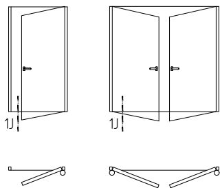
Сечение 1 – Нижний узел J.1 – Одностворчатые и двустворчатые французские двери. Нижний узел. Узкая створка АУРС.ВF73.0201 Открытие наружу *
