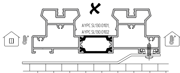
Схема обработки внутренней чашки профилей для установки винтов самонарезающих 3,9x13-A2ISO14585 для крепления монтажных пластин
