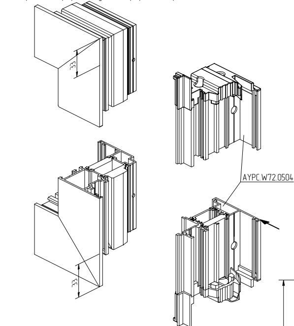
3. Установка штапикового комплекта фурнитуры ST (вариант 1), ST (вариант 2), 4005.03 Крепление профиля штапика к профилю створки
