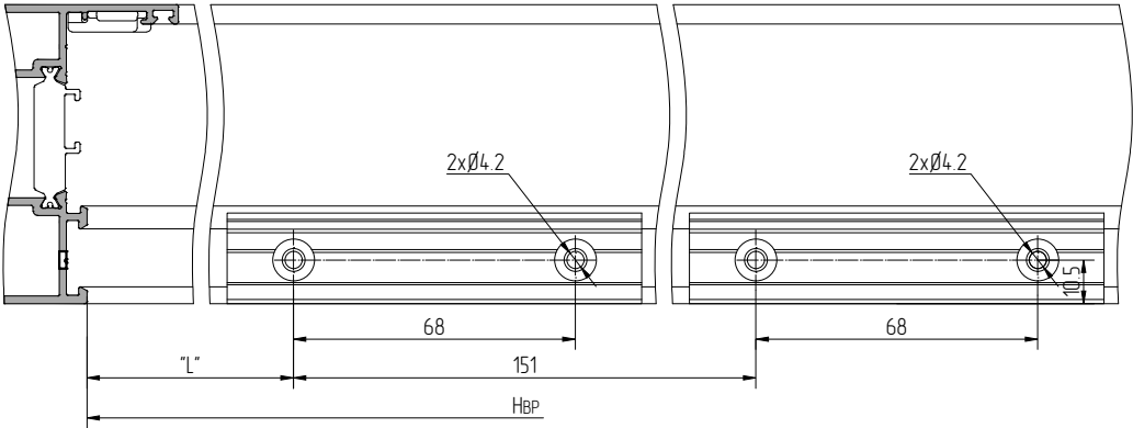
Обработка профиля рамы под установку 728940 с креплением 4,8х16-A2IS014586
