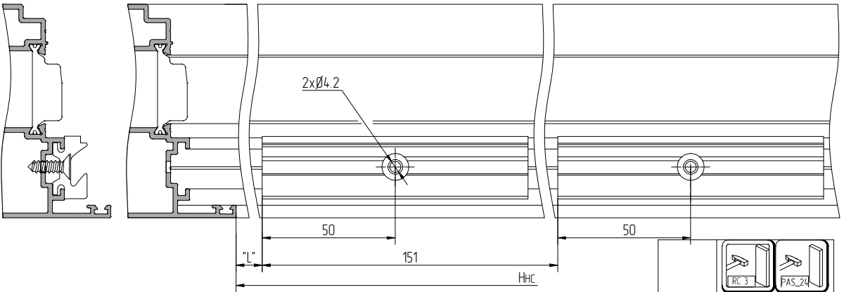
Обработка профиля створки под установку 728940 с креплением 4,8х16-A2IS014586
