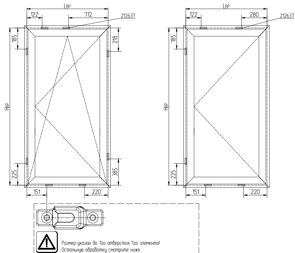
Схема установки 212637
