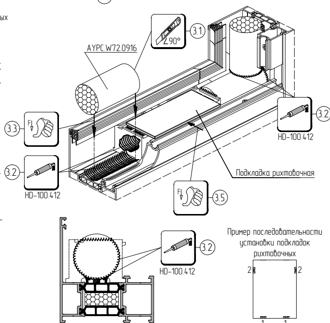
Схема нанесения герметика (операция 3.2)
