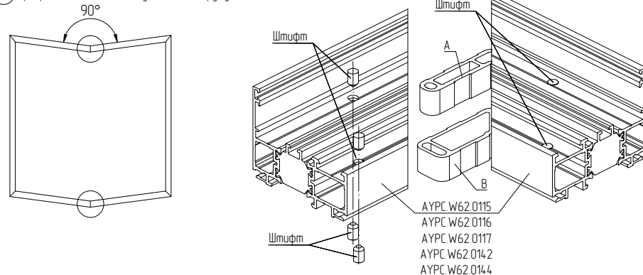
① Эркерный оконный блок с углом 90° наружу
