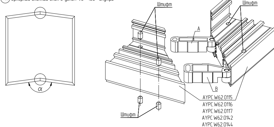
④ Эркерный оконный блок с углом 90°-180° внутрь
