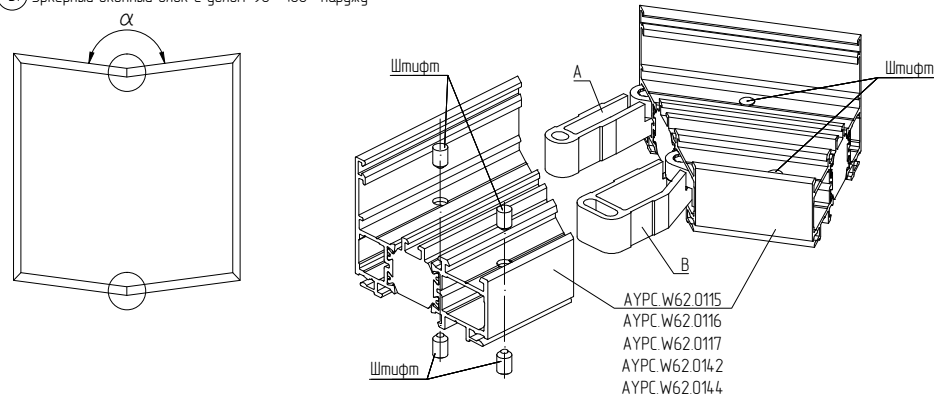
③ Эркерный оконный блок с углом 90°-180° наружу
