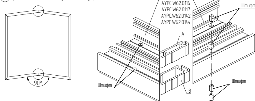
② Эркерный оконный блок с углом 90° внутрь
