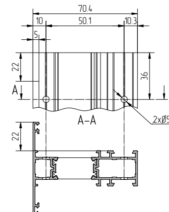
Схема обработки АУРС.W62.0321
