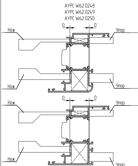
Обработка профиля для углового соединения методом обжима
