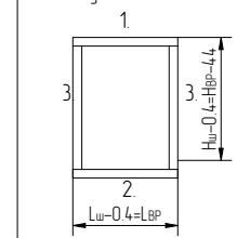
Схема установки штапика
