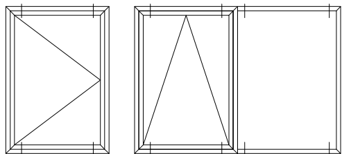
Противовзломные штапики
