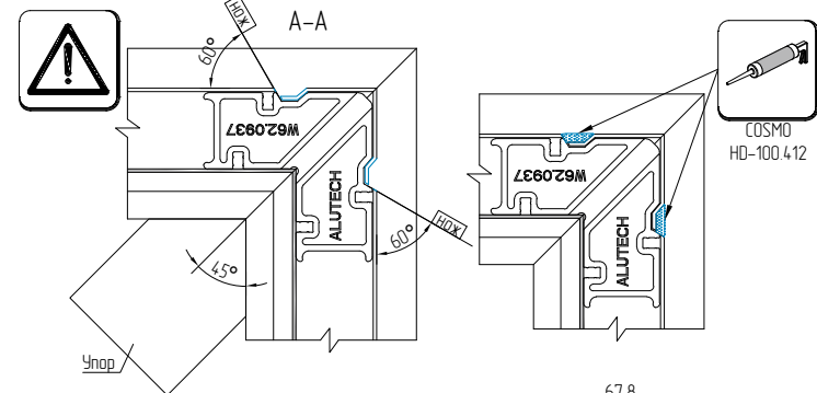
Данные для углового соединения методом обжима
