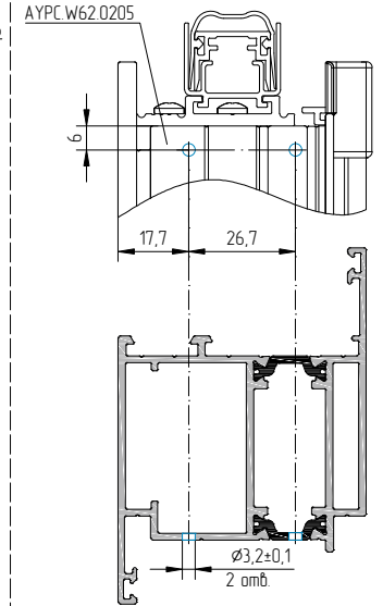
Схема обработки профиля створки AYPC.W62.0205 под установку манжеты EPDM AYPC.W62.0926
