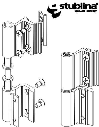
Петля STUBLINA арт. 2022.00
