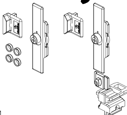
Комплект поворотного окна 4002.00
