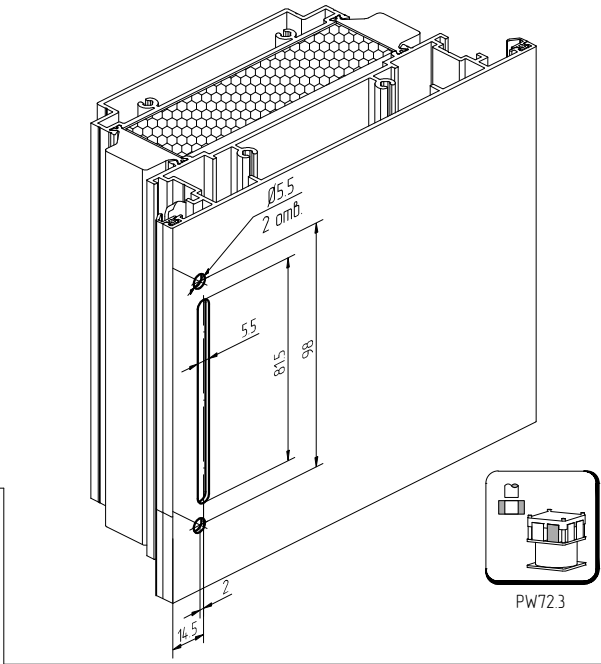
Схема обработки тяги АУРС.С48.0612 под фурнитуру STUBLINA
