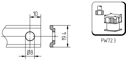
Схема обработки тяги АУРС.С48.0612 под фурнитуру STUBLINA
