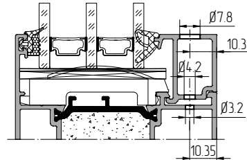
Схема крепления профиля штапика винтами самонарезающими 3,9x9,5-A2ISO14585
