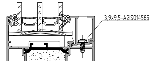
Схема крепления профиля штапика винтами самонарезающими 3,9x9,5-A2ISO14585
