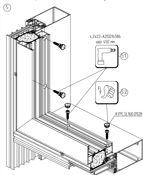
Схема крепления профиля спецрамы
