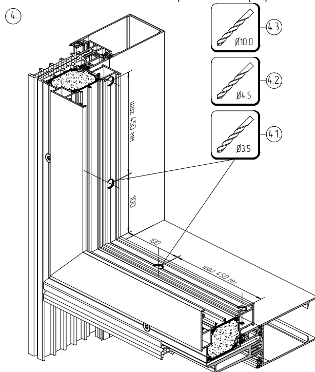
Схема обработки профиля спецрамы и профиля адгелтера
