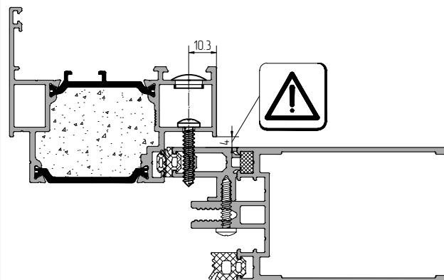
Схема крепления профиля спецрамы
