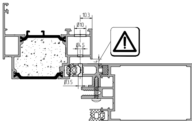
Схема обработки профиля спецрамы и профиля адгелтера
