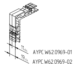
Закладные угловые из профиля AYPC.C48.0709
