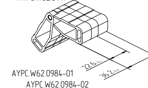
Закладная угловая из профиля AYPC.W62.0711
