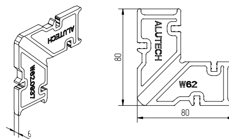
Закладная угловая литая AYPC.W62.0937
