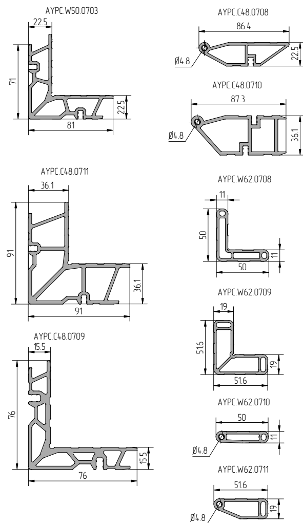
Закладная угловая из профиля AYPC.C48.0708
