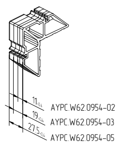
Закладная угловая из профиля AYPC.C48.0711
