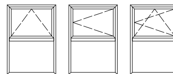
15. Двухстворчатое окно с горизонтальным импостом
