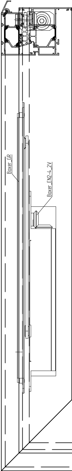
Схема установки доводчика скрытого GEZE Boxer_EN2-4_2V
