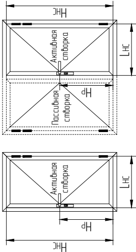
Исполнения дверной конструкции активной створки.
