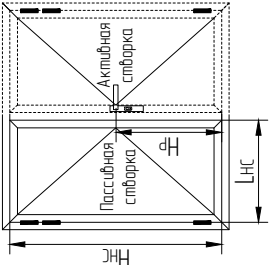
Исполнения дверной конструкции пассивной створки.
