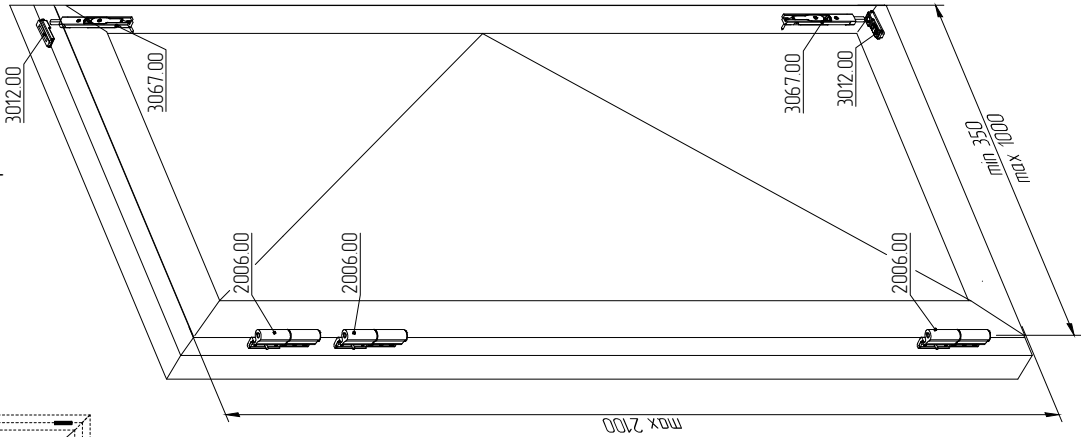
Исполнение 4 пассивная створка
