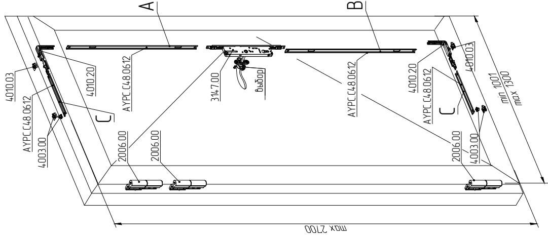
Исполнение 6 пассивная створка
