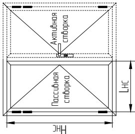
Исполнение 4 пассивная створка
