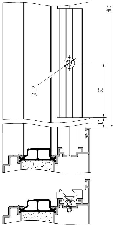
Обработка профиля створки под установку 728940 с креплением 4,8x16-A2ISO14,586
