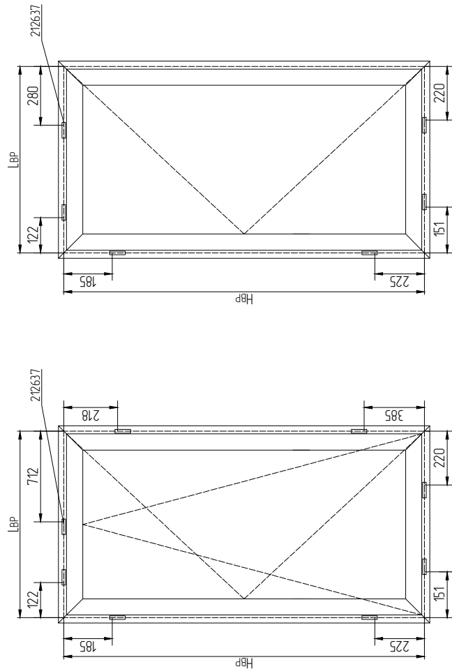
Схема установки 212637
