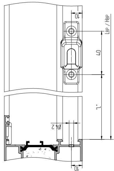
Обработка профиля рамы/импоста под установку 212637 с креплением 4,8х16-A2IS014586
