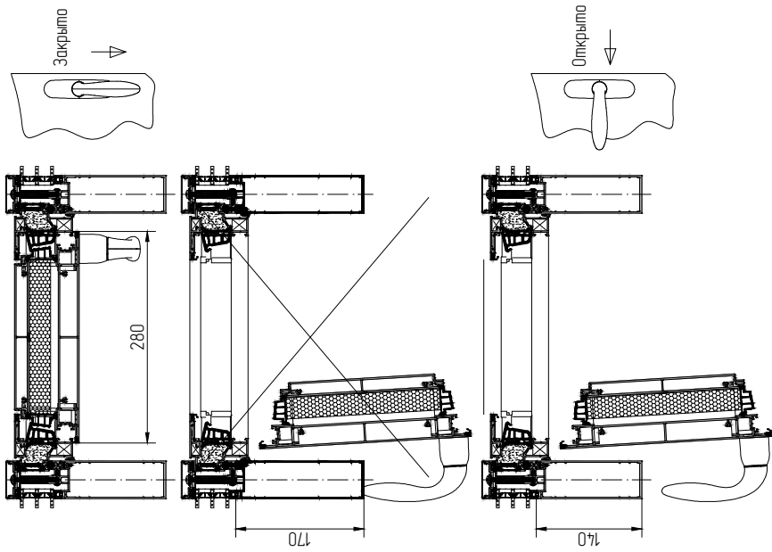
Варианты применения оконных ручек для вентиляционной створки
