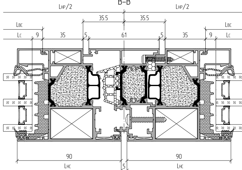
B-B
