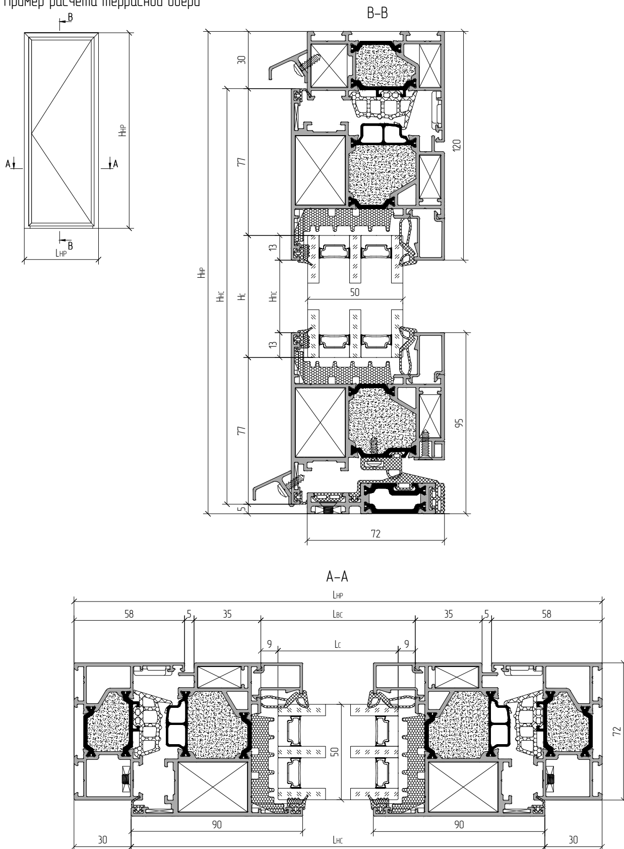
Пример расчета террасной двери
