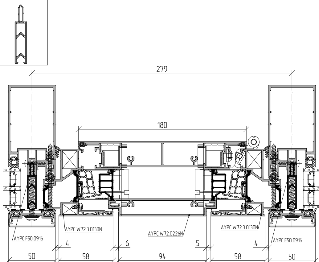
Исполнение 2
