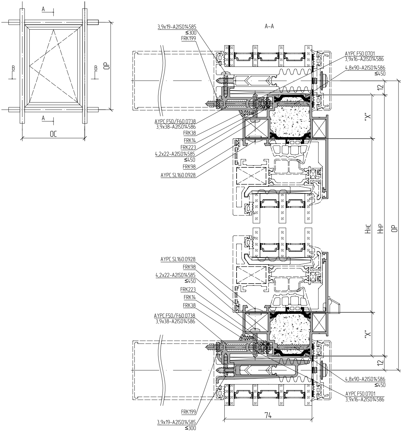
Пример расчета оконного блока с установкой в фасад
