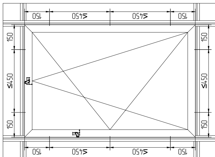
Обработка профилей АУРС.W72.3.0134, АУРС.W72.3.0135 и профиля АУРС.F50.0103 под 4.8x80-A2IS014586
