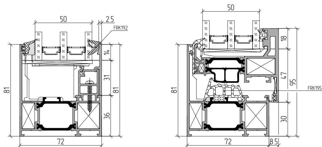
Исполнение 2
