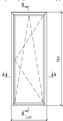
Пример расчета террасной двери
