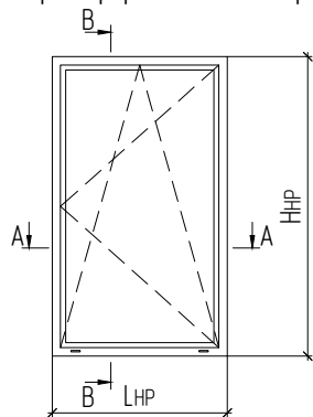
Пример расчета поворотно-откидного окна
