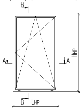
Пример расчета поворотного-откидного окна
