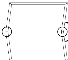
2. Эркёрный оконный блок с углом 90° внутрь
