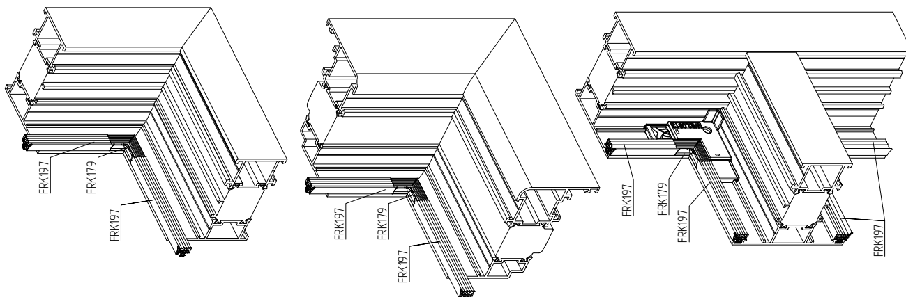
1) Установка FRK179
