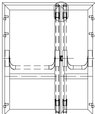
Пятиточечное запирание
