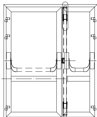
Трехточечное запирание
