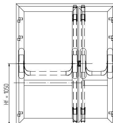
Пятиточечное запирание
