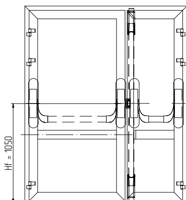
Трехточечное запирание
