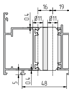
B-B AYPC.W72.0104
