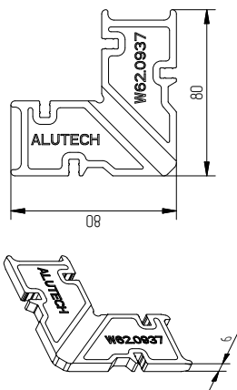
Закладная угловая литая АУРС W62 0937
