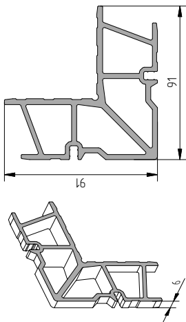
Закладная угловая экструдированная АУРС W62 0954-04
