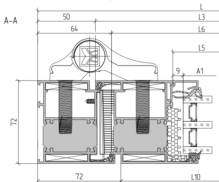
Пример расчета двуствольной двери открыванием внутрь
