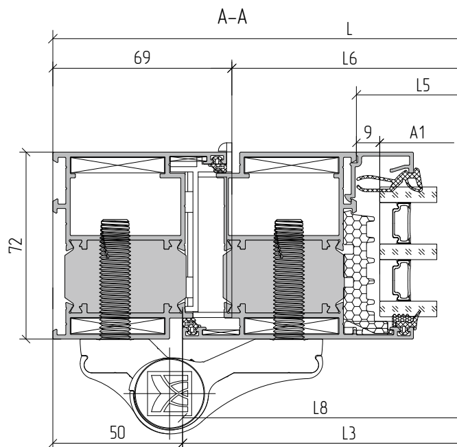
Пример расчета двупольной двери открыванием наружу
