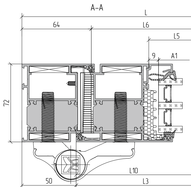
Пример расчета двуствольной двери открыванием наружу со штаплом
