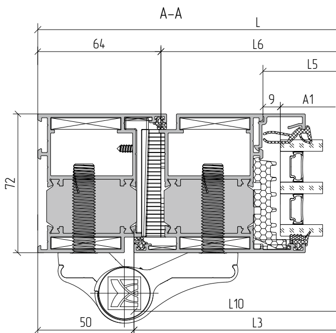
Пример расчета двупольной двери открыванием наружу
