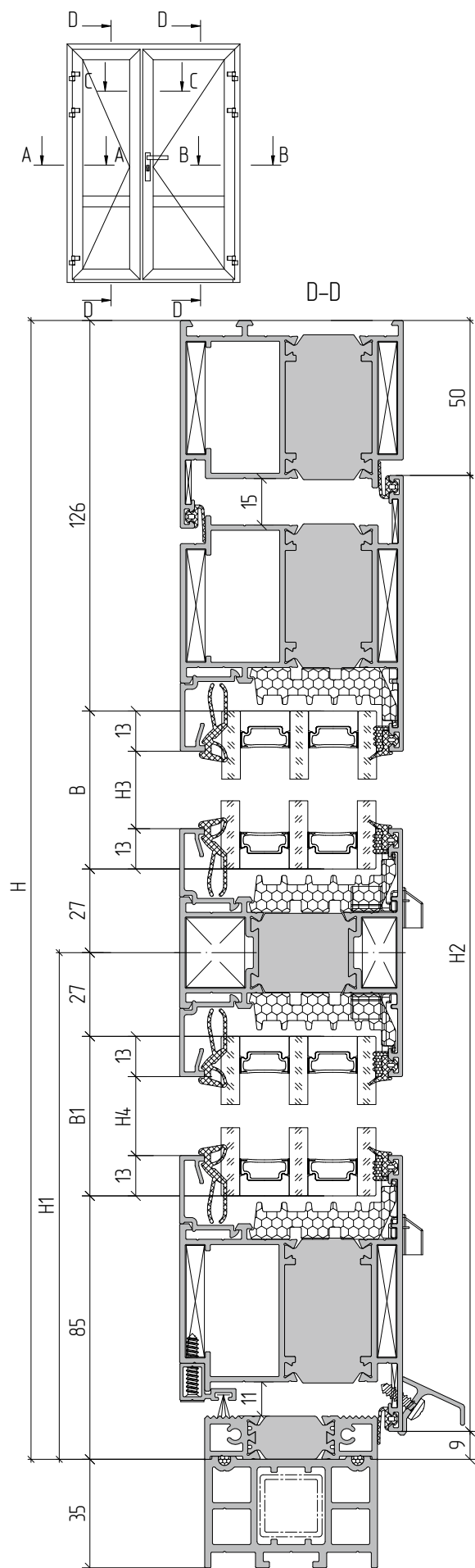
Пример расчета двупольной двери открыванием наружу
