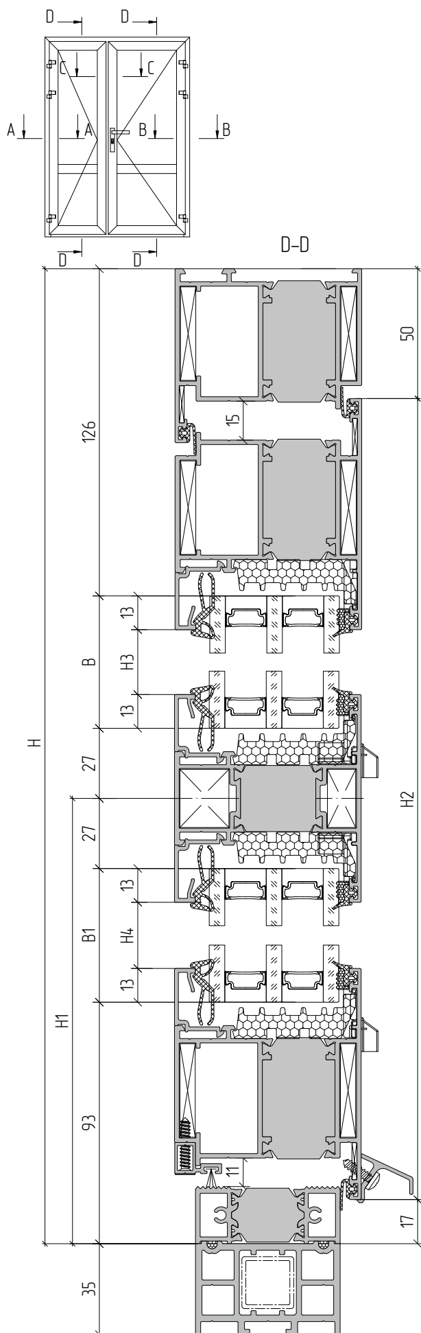
Пример расчета двустворчатой двери открыванием наружу
